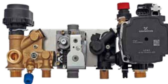
Grupo hidráulico
